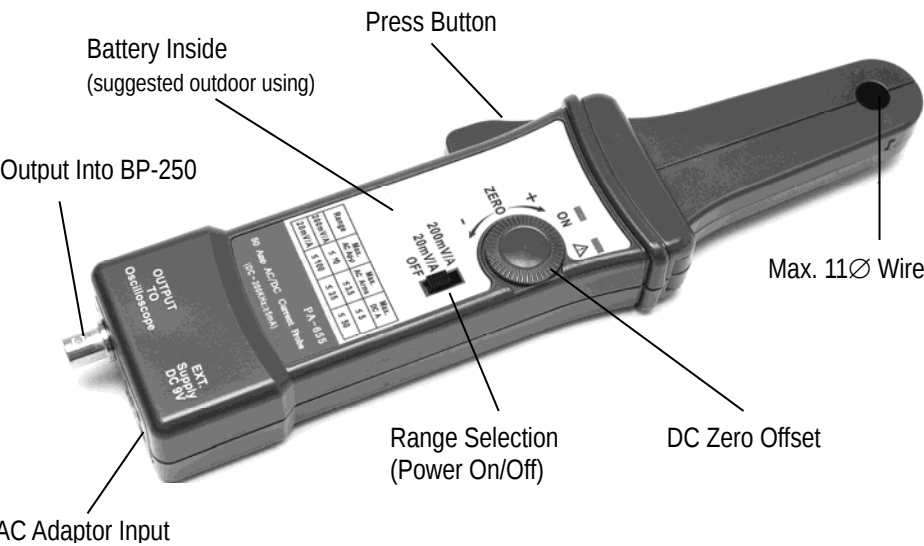
圖 1: PA-655 電流探測鉗上的控制及指示。
