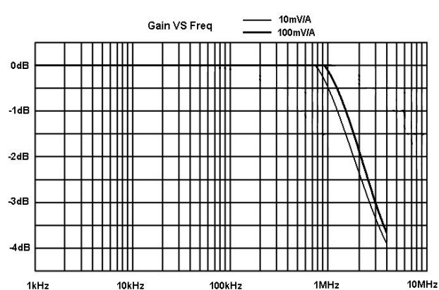
图 2 CPL8100D 典型增益频率关系曲线
